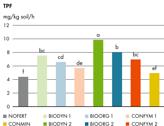
Figur 35: Dehydrogenaseaktivitet
